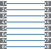
T568 A/B
